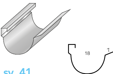
Canale Tipo B SV. 41
