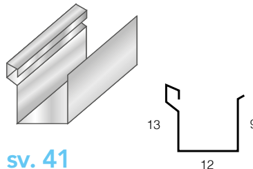
Canale Tipo M SV. 41 + aletta 1 cm
