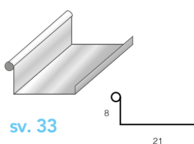
Scossalina Tipo C SV. 33
