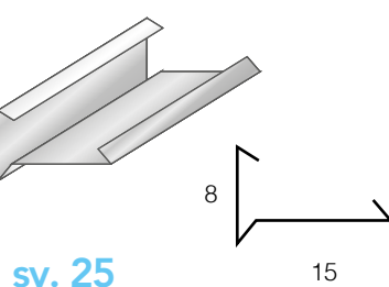
Scossalina Teramo SV. 25
