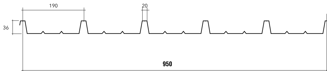
PROFILO 5 GRECHE: A38D760G5
