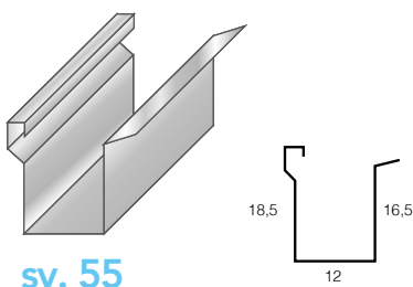
Canale Tipo S SV. 55 - Alto
