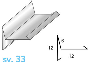
Scossalina "T" 35 SV. 33 - Aperta
