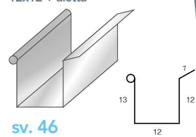
Canale Quadro 12x12 + aletta
