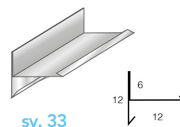
Scossalina "T" SV. 33 - Schiacciata
