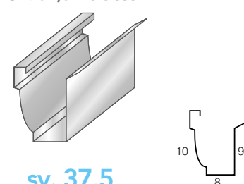
Canale Tipo A SV. 37,5 ridotto
