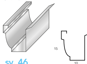
Canale Tipo A SV. 46
