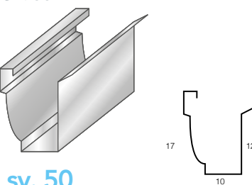
Canale Tipo A SV. 50
