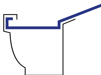
Esempio di gronda con sostegno interno
