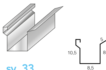
Canale Tipo S SV. 33 - ridotto + aletta
