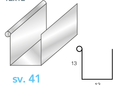
Canale Quadro 12x12
