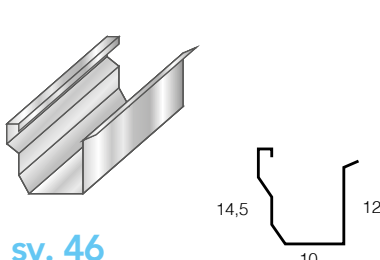
Canale Tipo Puglia SV. 46
