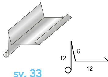
Scossalina "T" 36 SV. 33 - Aperta con riccio
