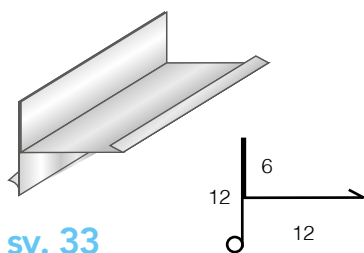
Scossalina "T" 34 SV. 33 - Schiacciata con riccio
