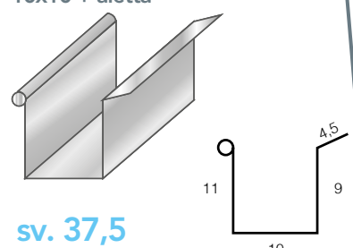
Canale Quadro 10x10 + aletta
